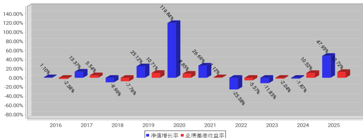
工银新趋势灵活配置混合C基金每年净值增长率与同期业绩比较基准收益率的对比图（2025年12月31日）
